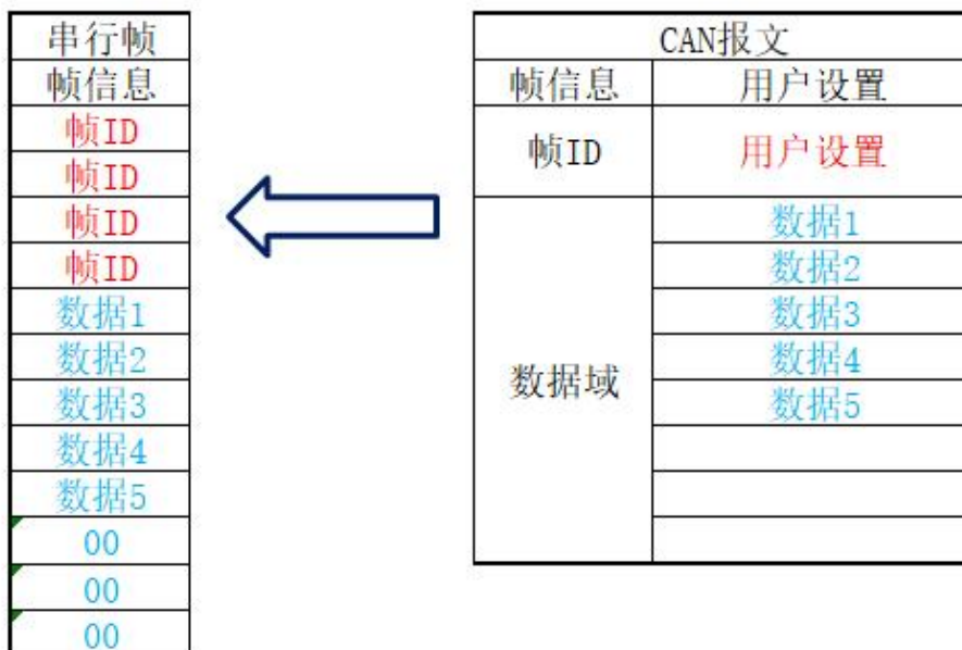
图 4.7 CAN 报文转串行帧（透明带信息转换）
