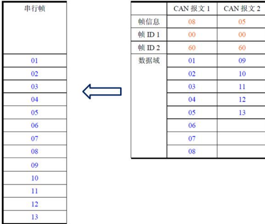
图 4.4 CAN 报文转串行帧示例（透明转换）
