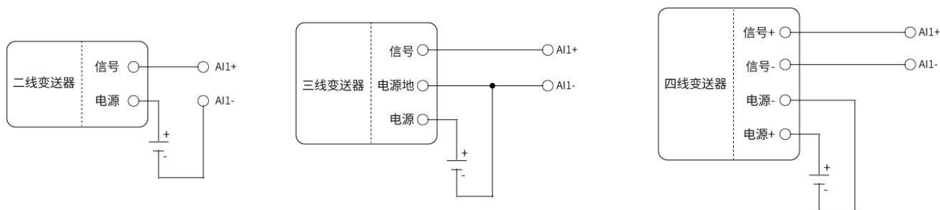
模拟量输入连接
