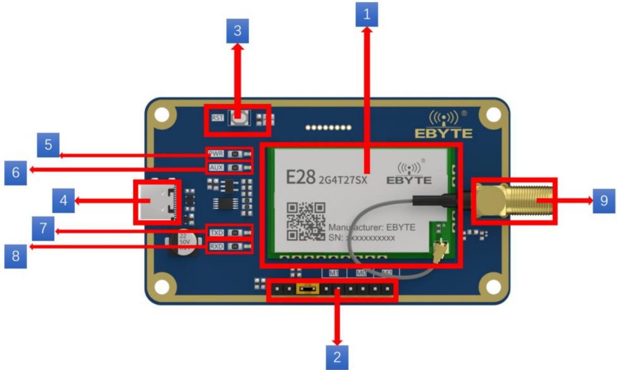
图 2 部件分布图
