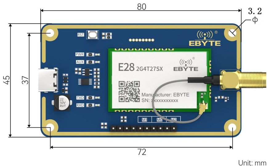
图 3 尺寸图
