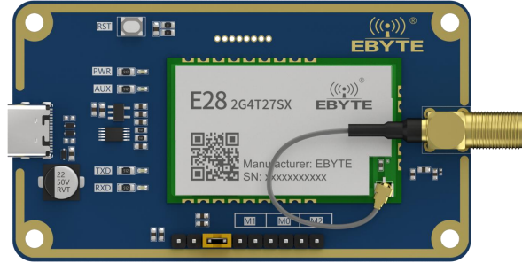
图 1 产品外观图
