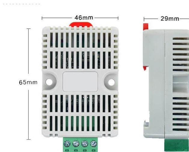
图 1-1 产品尺寸图
