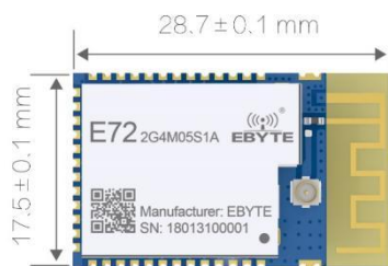
E72-2G4M05S1A
