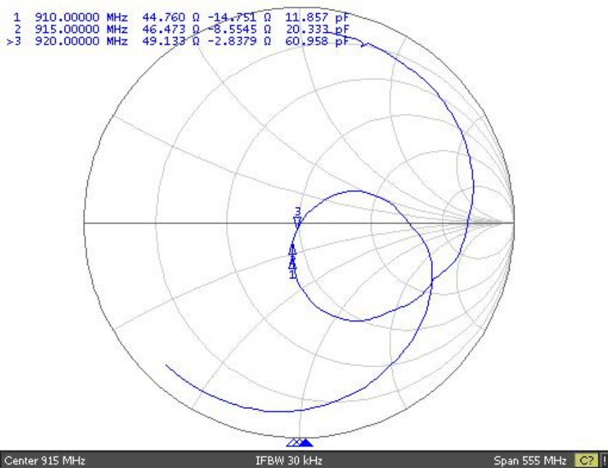
史密斯圆图 (Smith chart)
