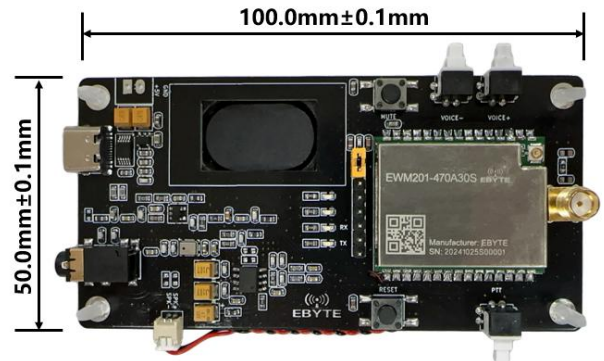
图 2: EWT201-470A30S
