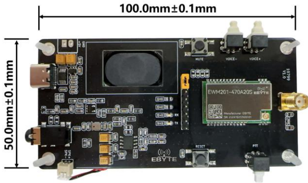
图 1: EWT201-470A20S
