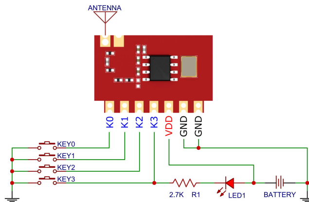
E160-TxFS1 参考电路
