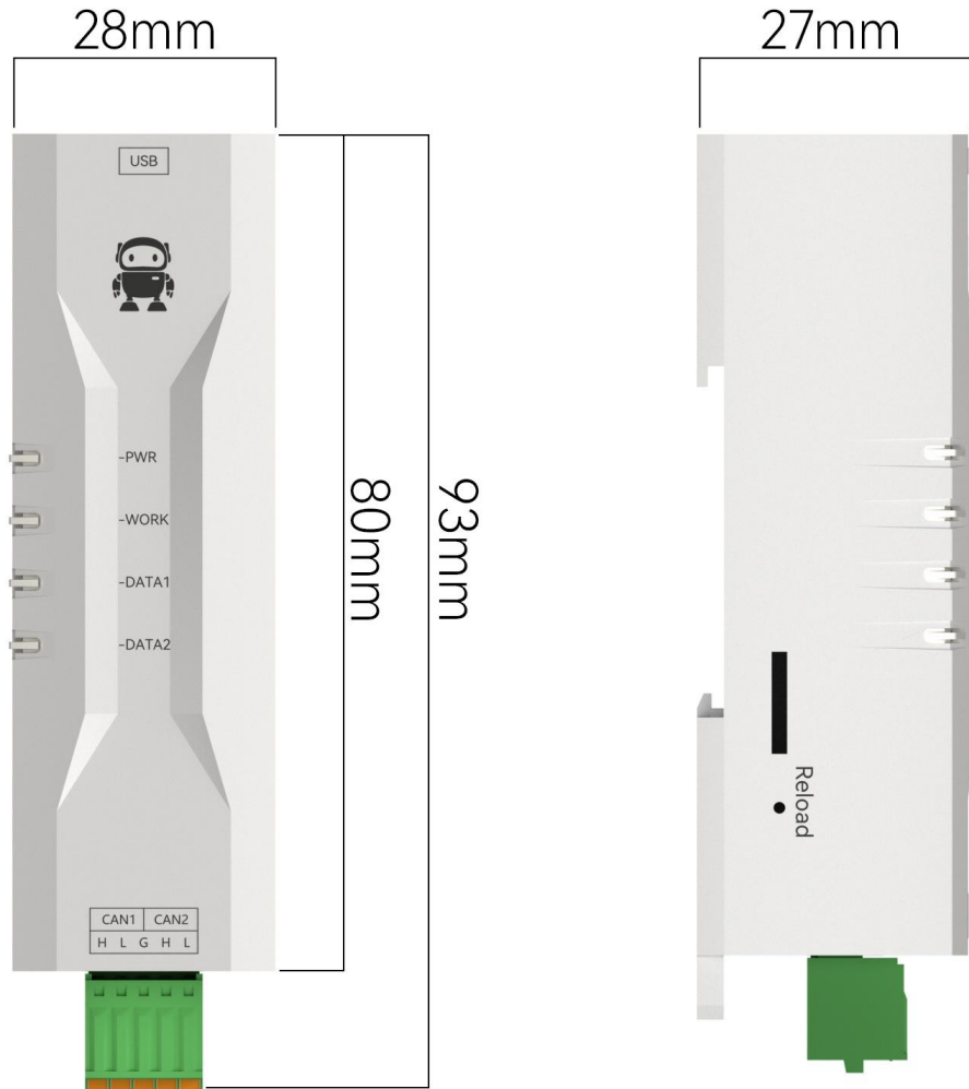
图 2.1 ECAN-U01M/ECAN-U01MS 外形尺寸
