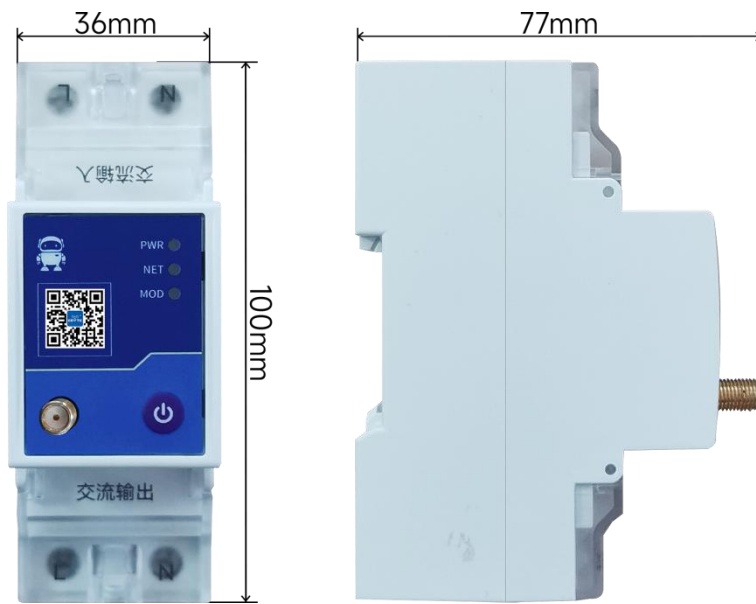
CE31-K02T 尺寸图
