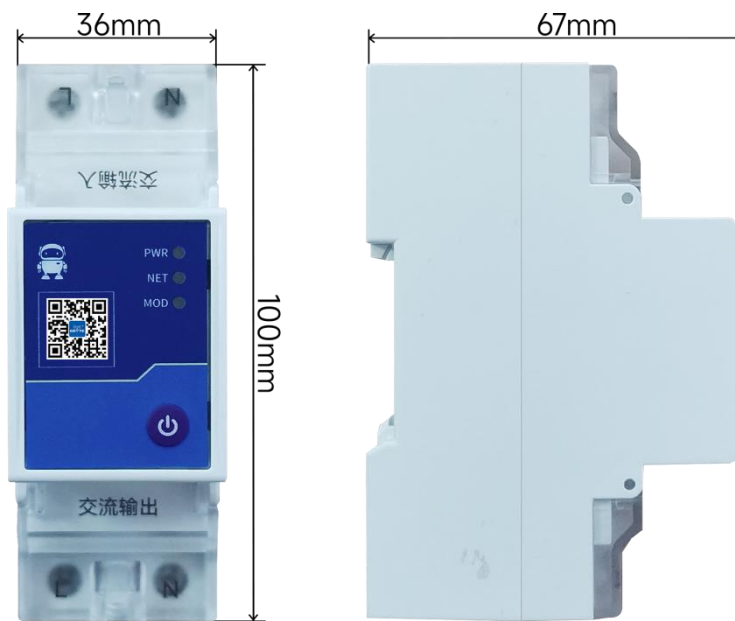
CE31-K02 尺寸图
