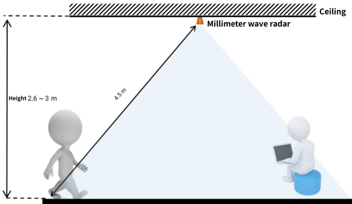
图 6-1 挂顶安装示意图
