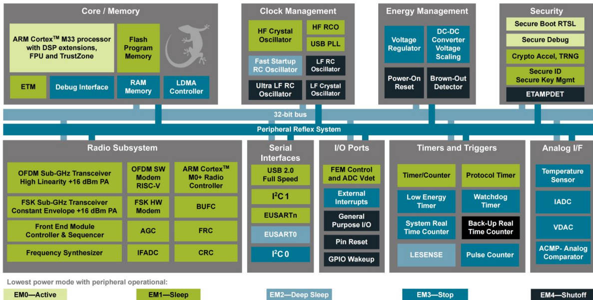
EFR32FG25 系列芯片内部功能框图
