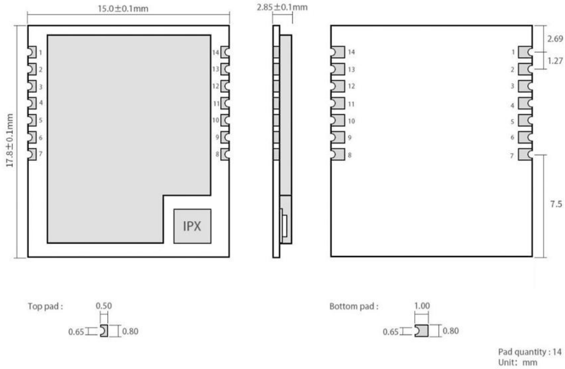
E28-2G4M12SX 机械尺寸
