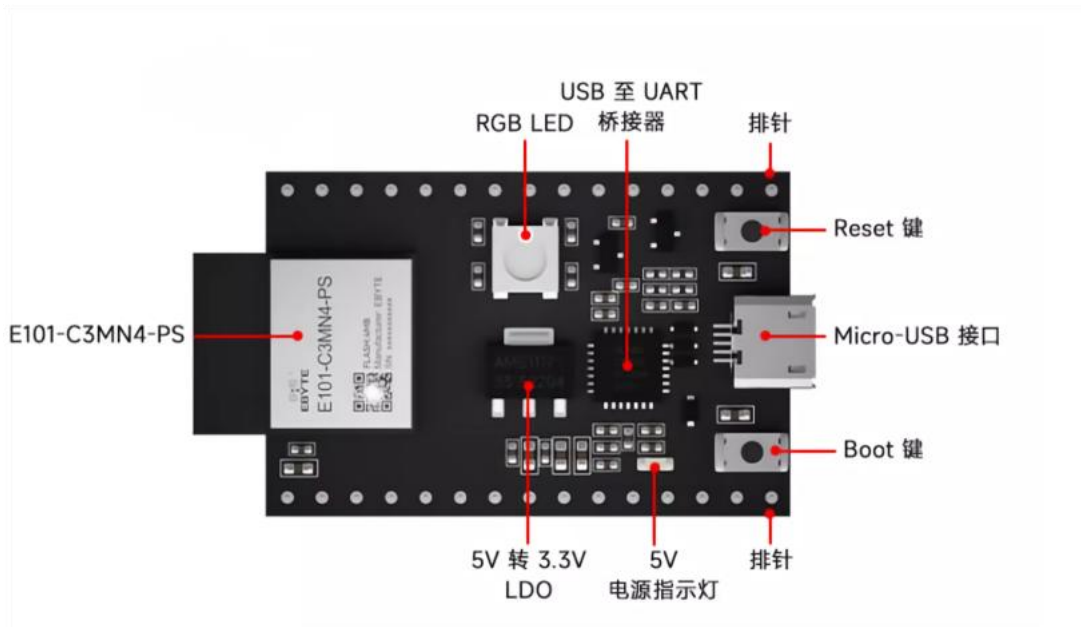
图一 主要组件图以 E101-C3MN4-PS-TB 为例
