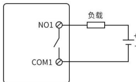
DO 输出连接示意图
