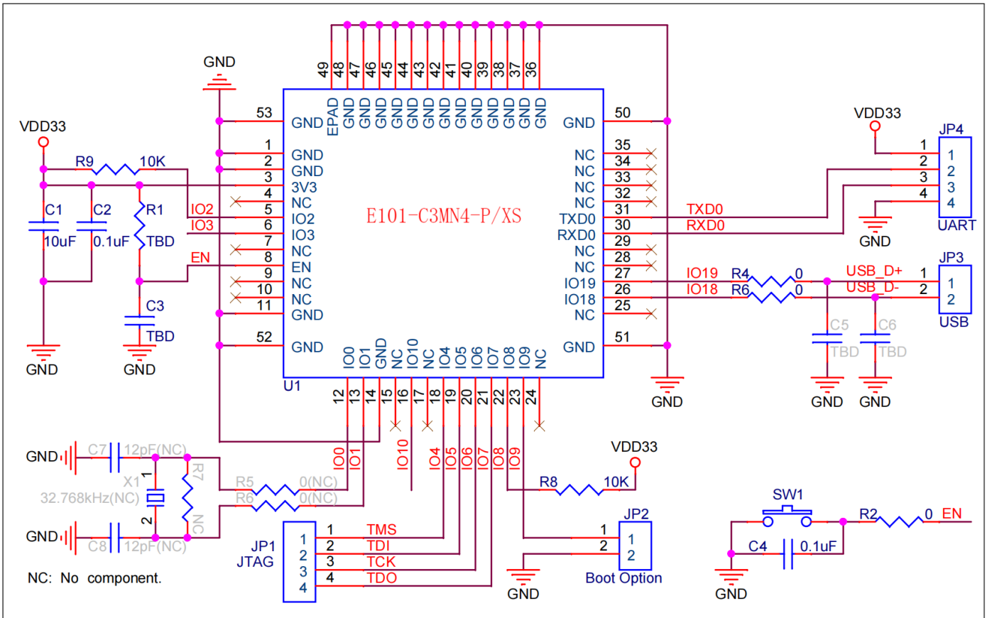
图表 0-3 推荐原理图
