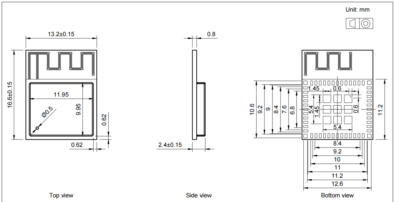
图表 0-5 模组尺寸
