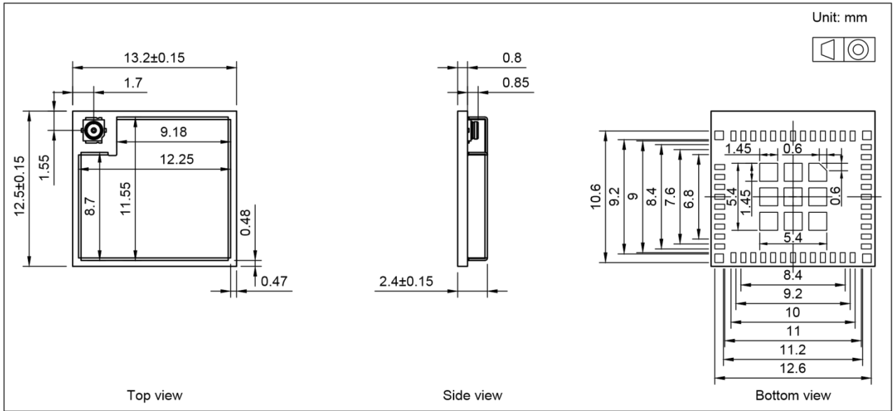
图表 0-4 模组尺寸
