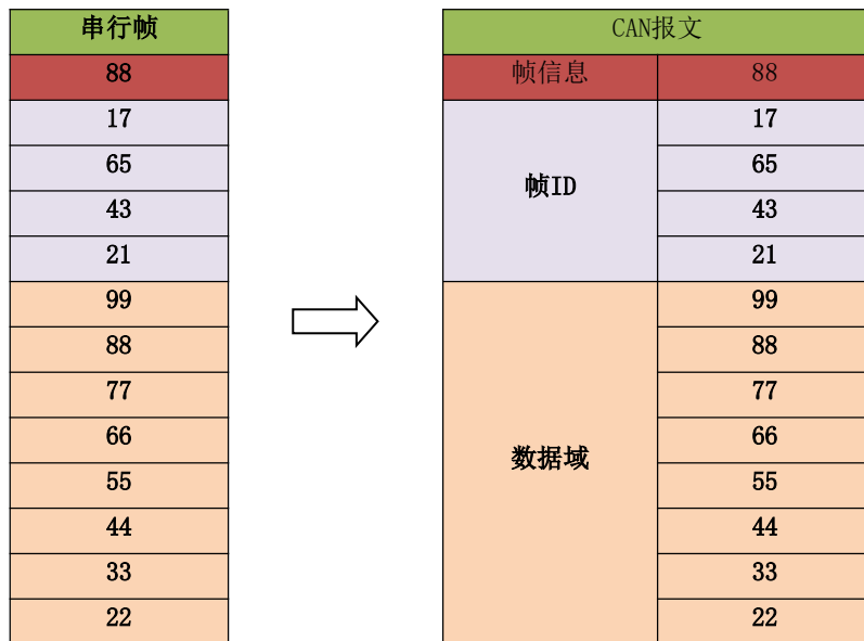
串行帧转CAN报文（协议模式）
