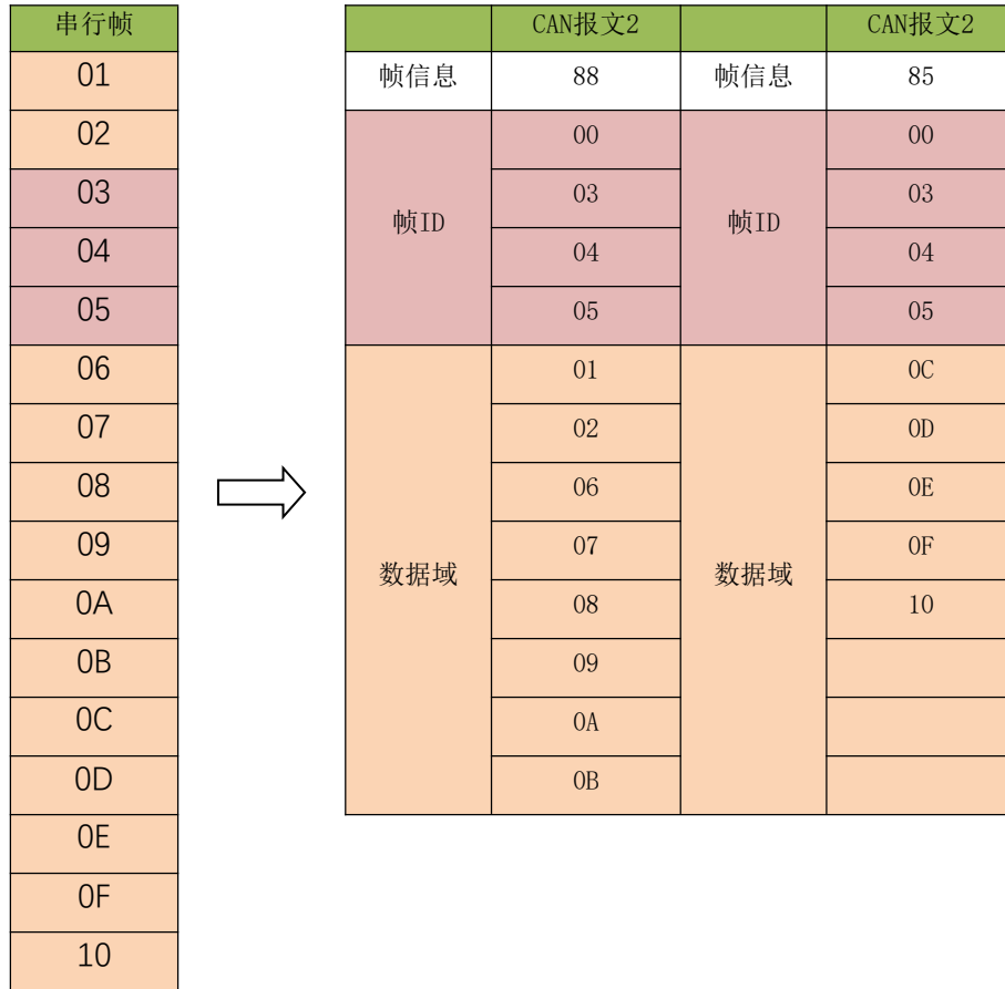
串行帧转 CAN 报文示例（透传带标识转换）
