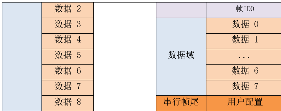
CAN报文转换成串行帧
