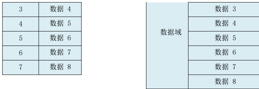
串行帧转换成 CAN 报文（透明方式）
