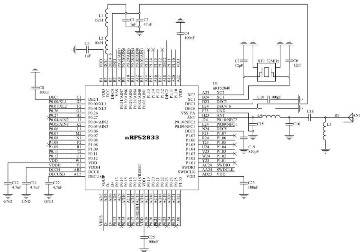
图 5-1 电路图
