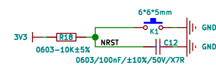
复位设置电路
