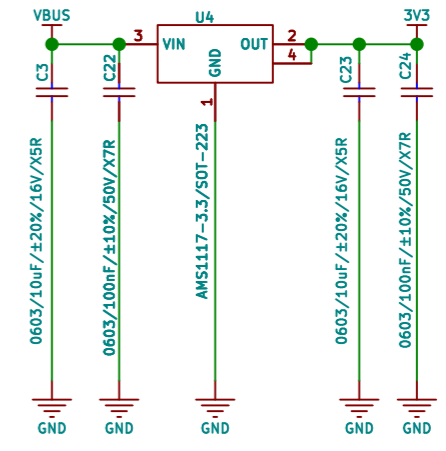
LDO电路
