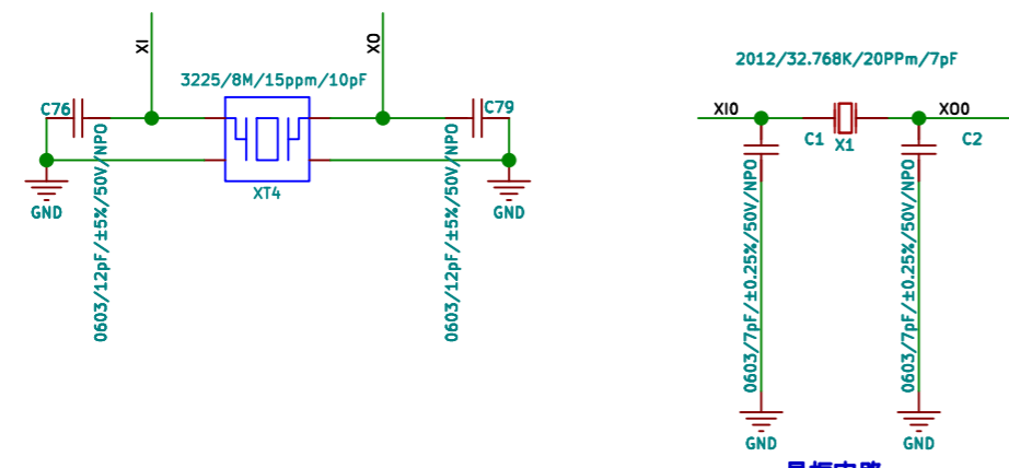
晶振电路
