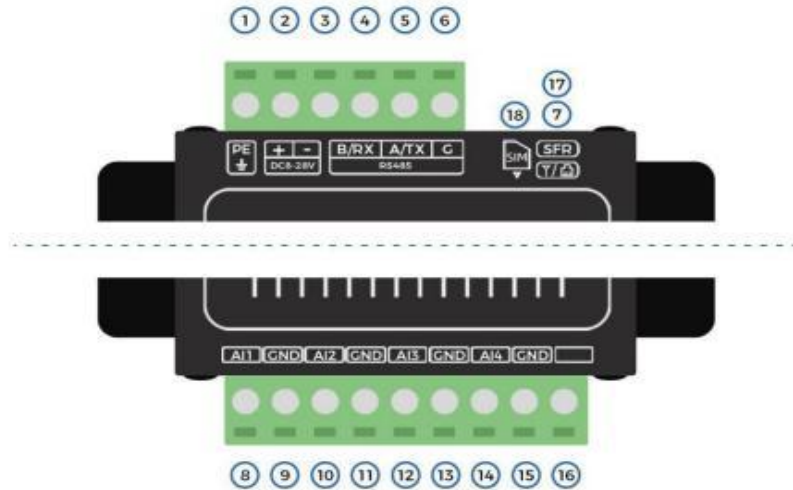
图 1-3 发送（采集）端产品接口展示
