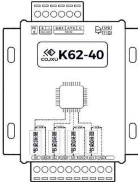
模拟量输入产品内部原理简图
