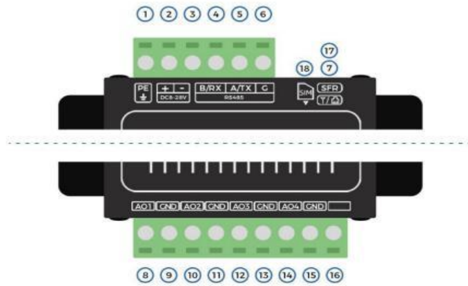
图 1-4 接收（输出）端产品接口展示
