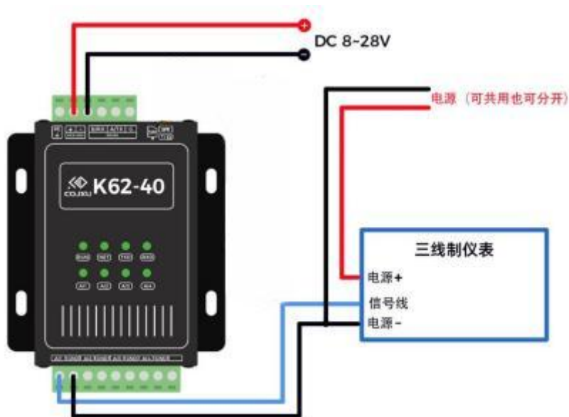
图 3-3 三线制接线图
