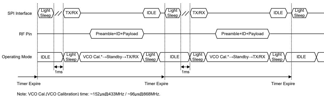
周期性 TX/RX 时序
