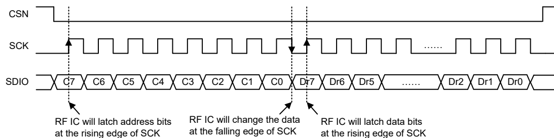
3 线 SPI 接口读取 1 个字节数据
