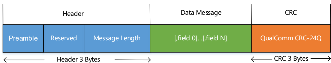
图 4-1 RTCM 帧结构
