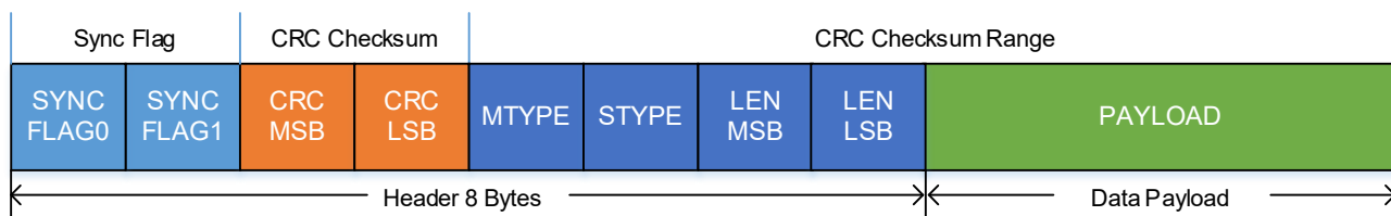
图 3-1 BK 帧结构
