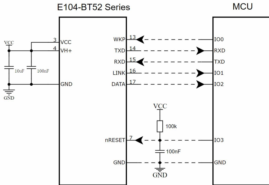
图 4-1 推荐电路
