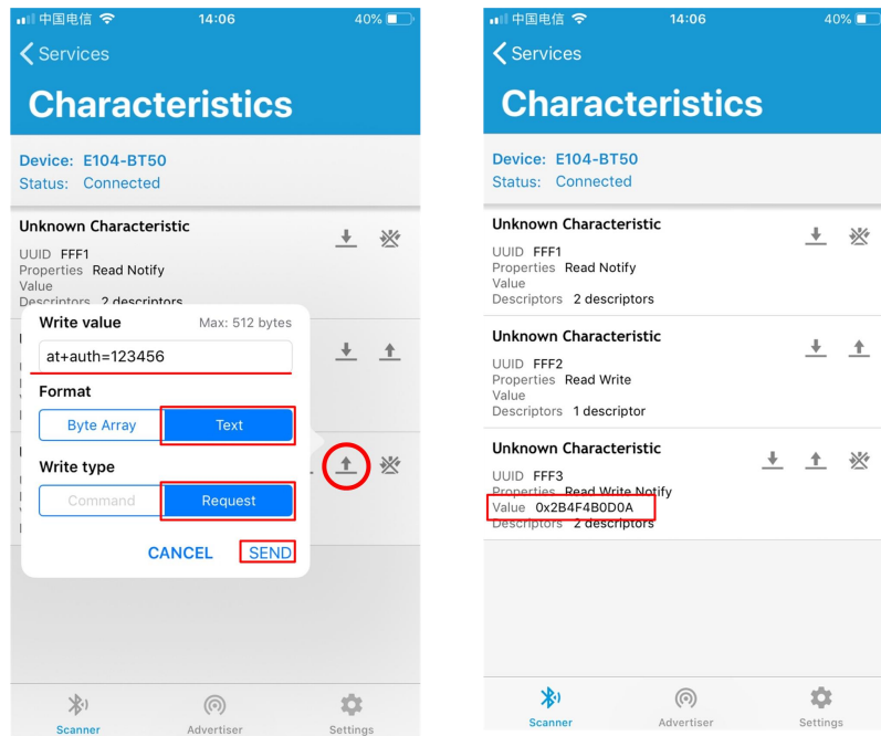
图表 七- 4 空中配置认证图
