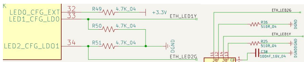
网络 LED 配置及外接指示灯参考电路图
