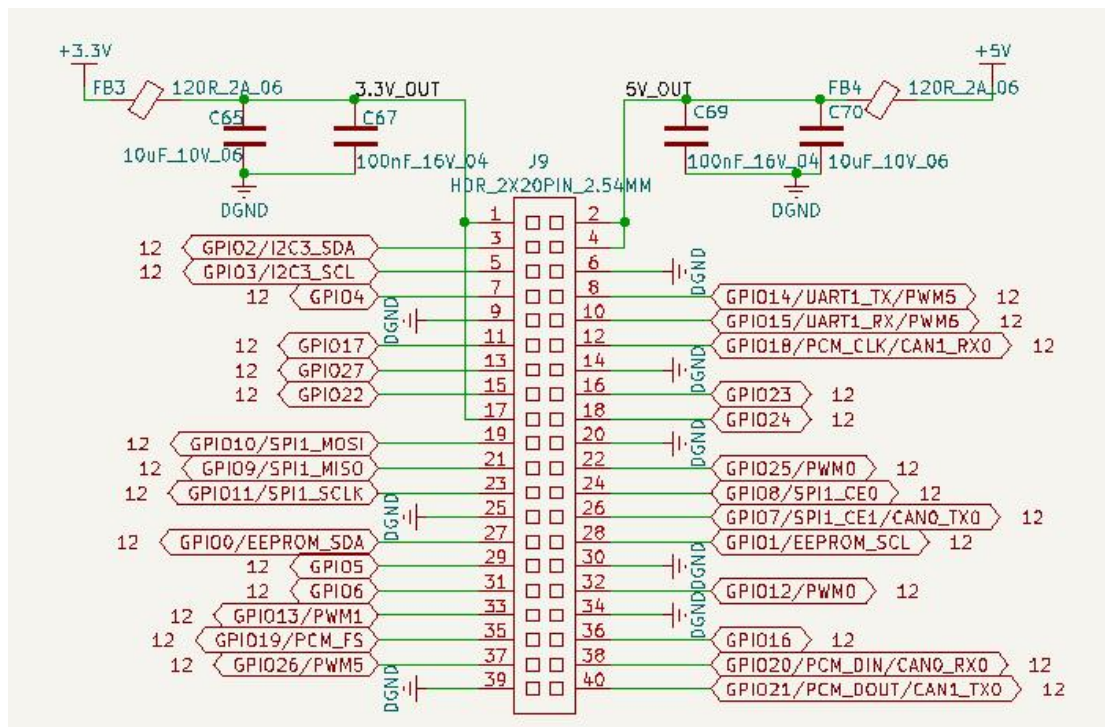
树莓派 2*20 接口电路示意图
