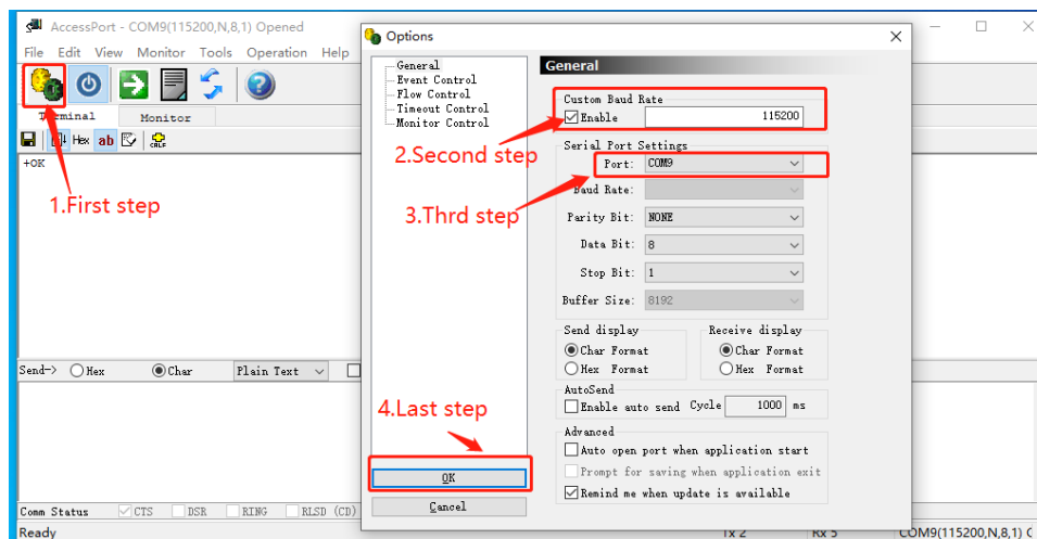
图表 4-1-2 AccessPort 参数配置,其他参数默认
