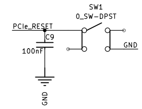
按键复位
