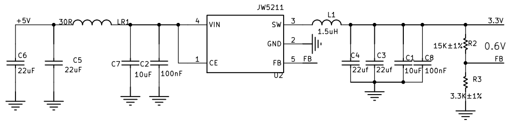
电源转换
