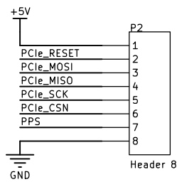
排针接口
