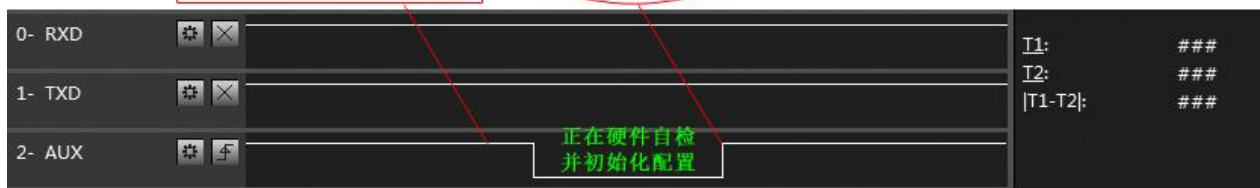
自检期间，AUX引脚时序图
