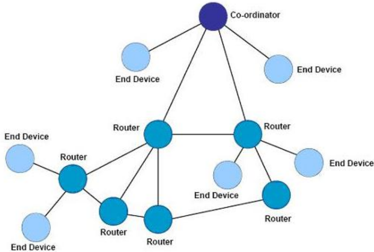
网络结构图
