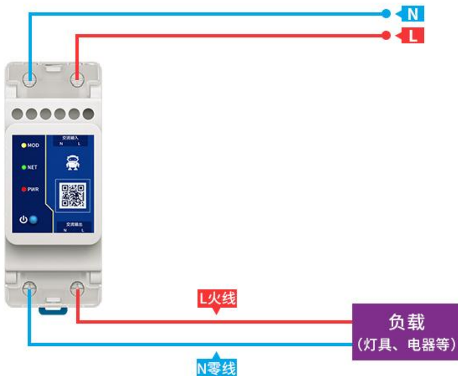
CE31-K01接线图
