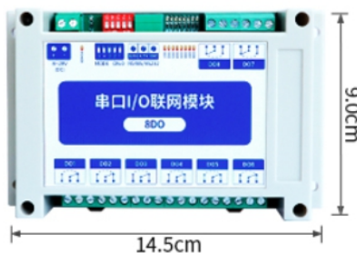
8路开关输出
