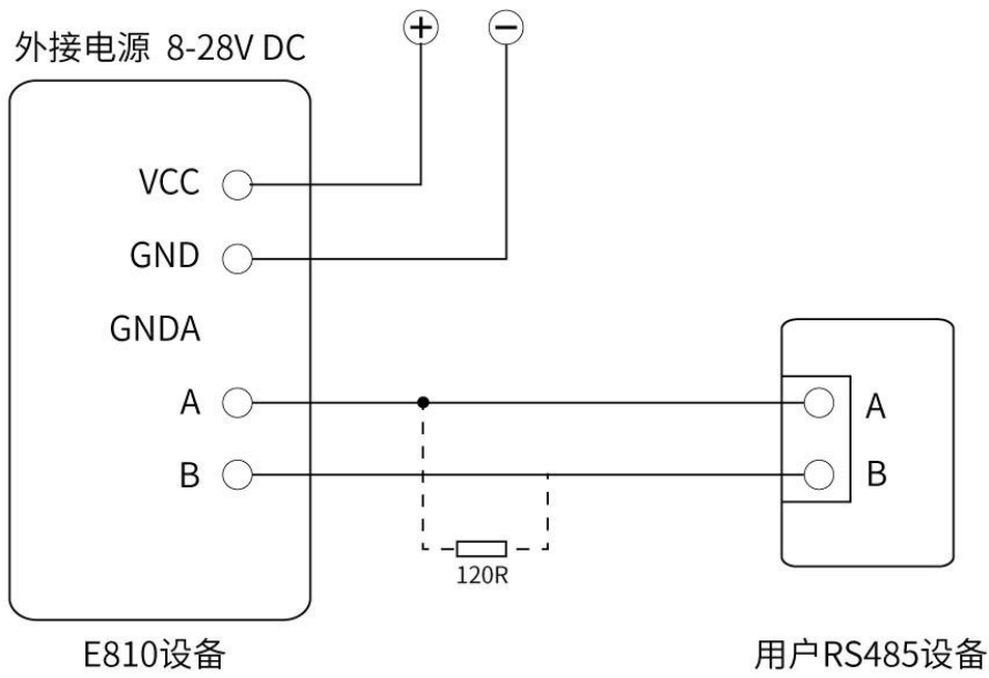
RS485接线图
